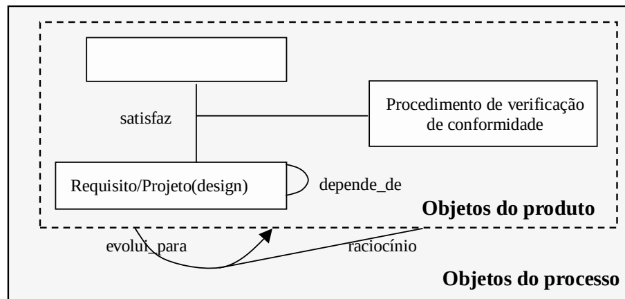
Figura 7: Meta-modelo de rastreamento de Ramesh
