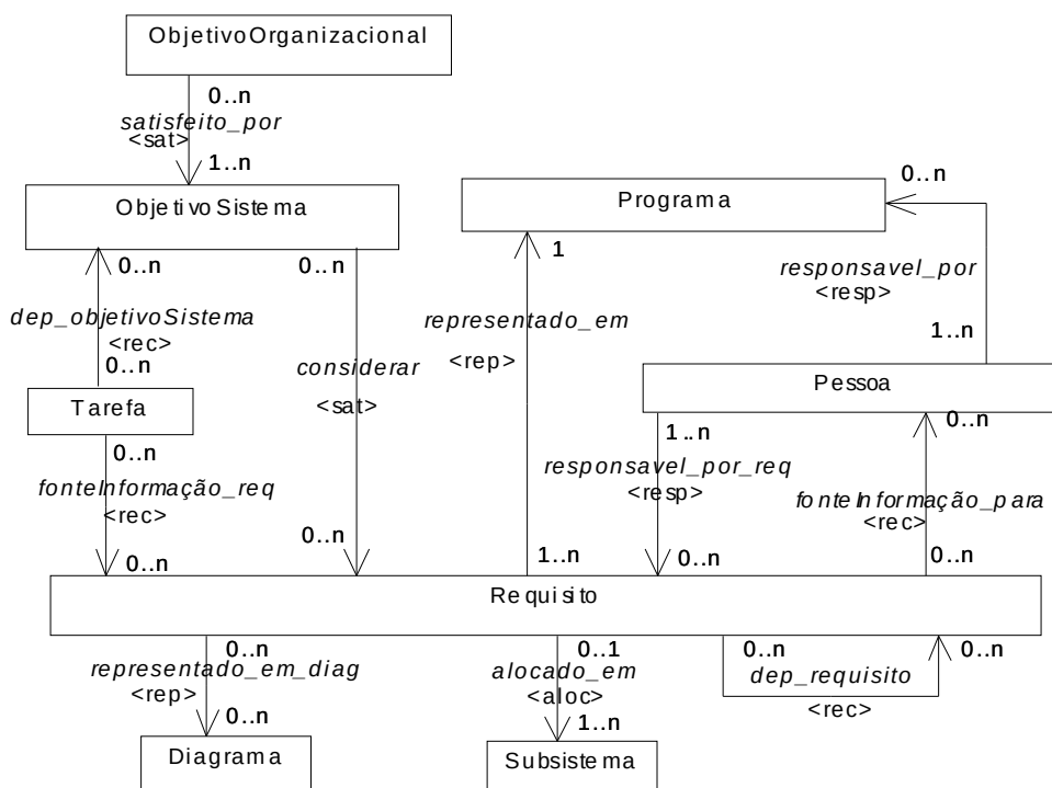
Figura 57: Modelo de rastreamento do sistema de controle de locadora
