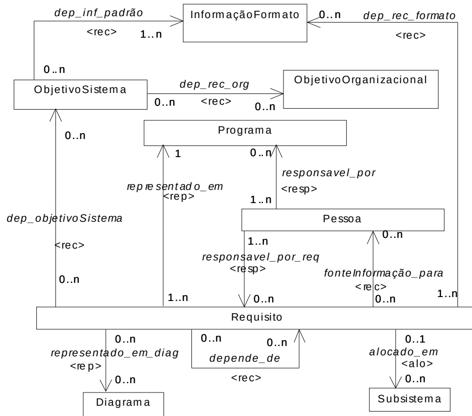
Figura 74: Modelo de rastreamento do sistema de biblioteca
