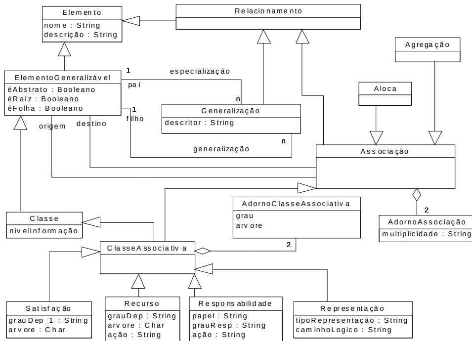
Figura 15: Meta-modelo para o rastreamento
