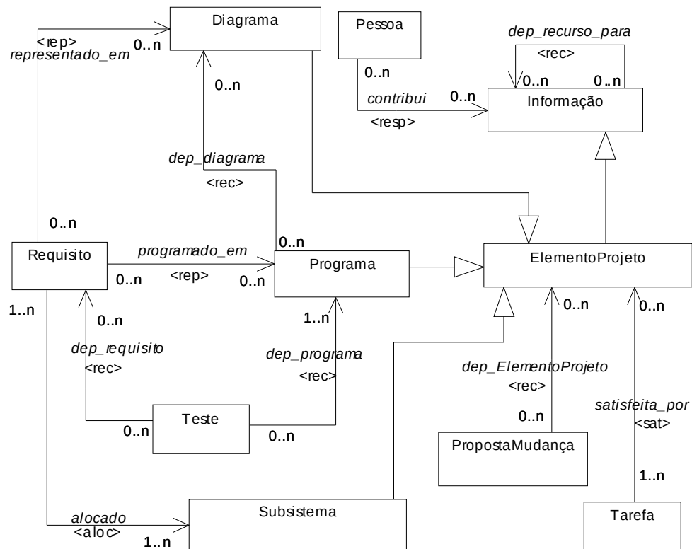
Figura 39: Sub-modelo de rastreamento para o projeto de software
