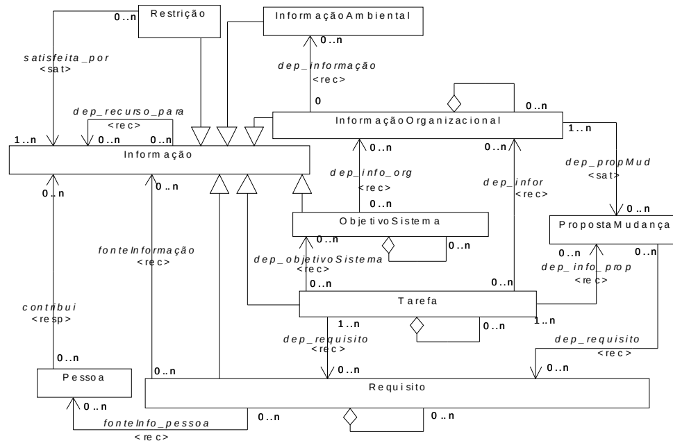
Figura 38: Sub-modelo para a gerência de requisitos
