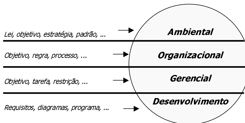
Figura 13: Classificação da informação do rastreamento
