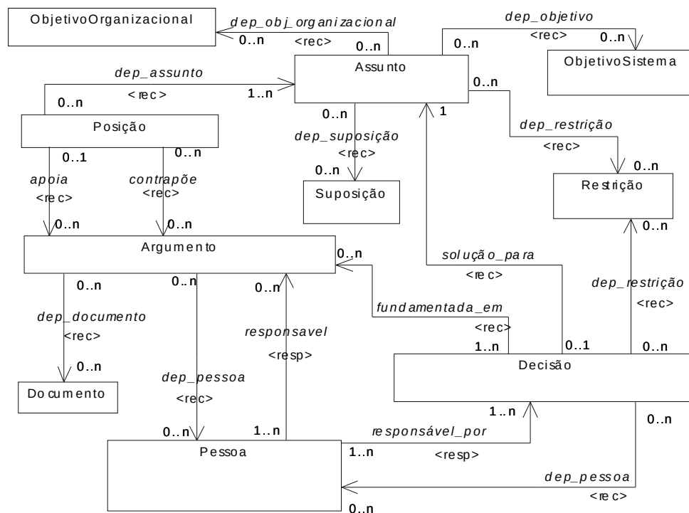
Figura 40: Sub-modelo para o raciocínio
