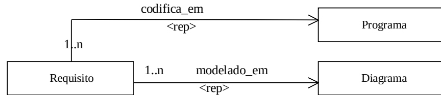
Figura 31: Representação da associação representação
