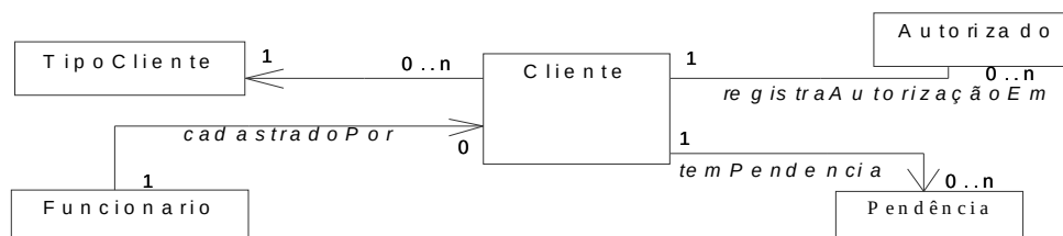
Figura 52: Diagrama de classe sobre a classe cliente
