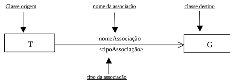
Figura 16: Alguns elementos básicos de uma associação
