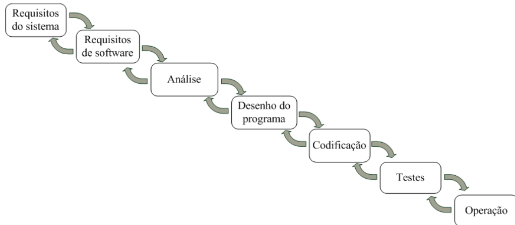
Figura 4-1 – Modelo Cascata
