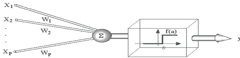
Figura 3.1: Neurônio de McCulloch e Pitts (1943).
