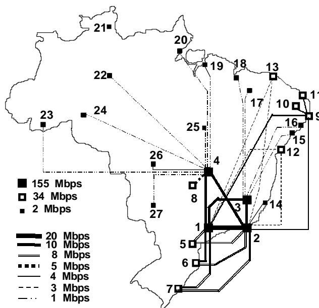
Figura 3 – Topologia de simulação
