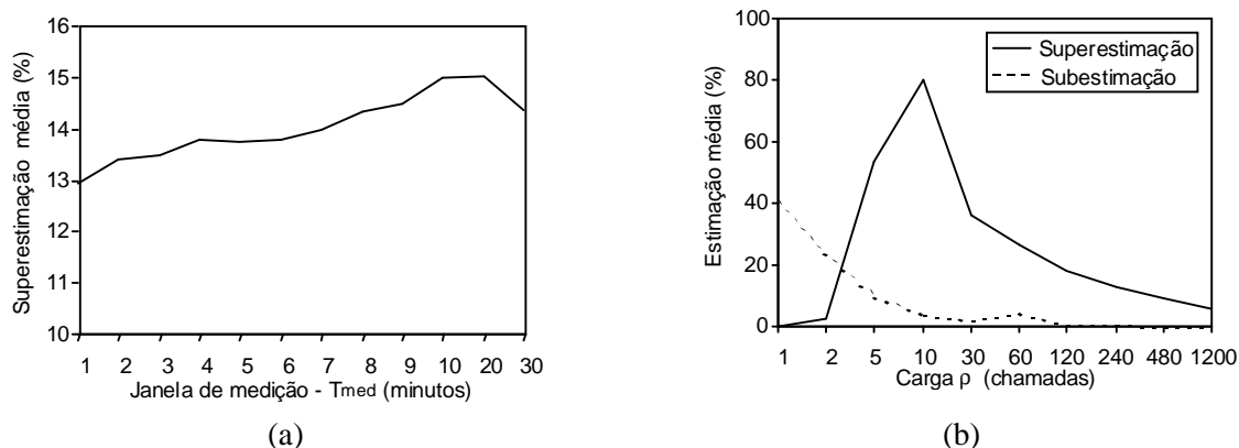
Figura 5 – Efetividade das estimativas; a) superestimação em relação à janela de medição T_{med} ; b) superestimação e subestimação em relação à carga \rho .
