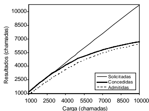
Figura 8 – Chamadas geradas, solicitadas, concedidas e admitidas no sistema
