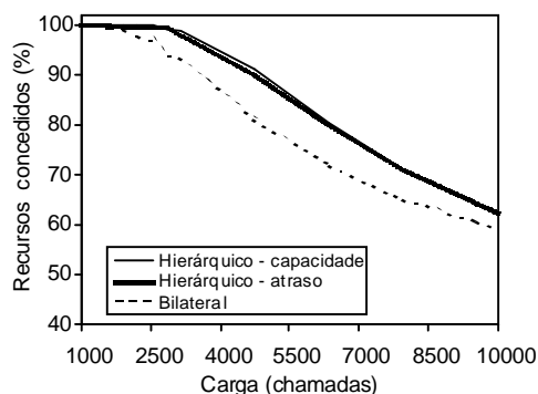
Figura 6 – Recursos concedidos com relação à carga do sistema
