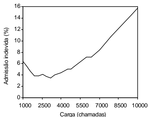
Figura 9 – Chamadas admitidas indevidamente
