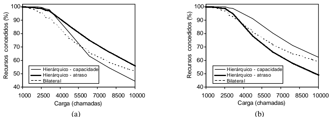
Figura 7 – Recursos concedidos com alterações nas configurações; a) capacidade do enlace 1-2 alterada para 5 Mbps; b) atraso do enlace 1-2 alterado para 50 ms.
