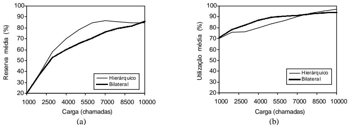
Figura 10 – Provisionamento e utilização de recursos; a) percentual de recursos reservados em relação ao disponível; b) percentual de recursos utilizados em relação ao reservado.
