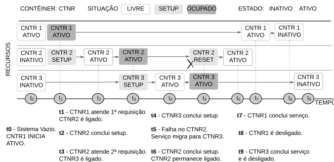
Fig. 2. Exemplo de operação para n = 1 , c = 3 e k = 3 .
