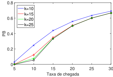
(a) Probabilidade de bloqueio (PB)
