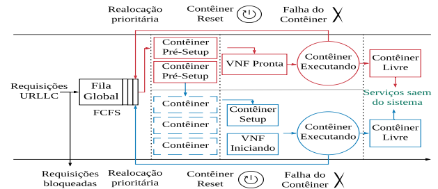
Fig. 1. Sistema URLLC MEC-NFV.
