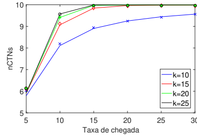
(b) Número médio de contêineres inicializados (nCTNs).
