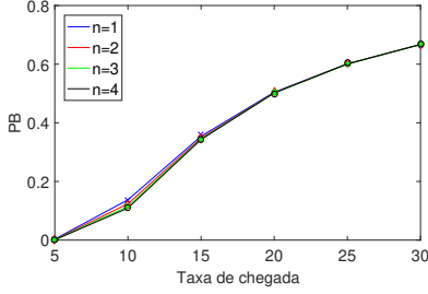
(a) Probabilidade de bloqueio (PB)
