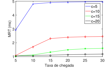
(c) Tempo médio de resposta (MRT).
