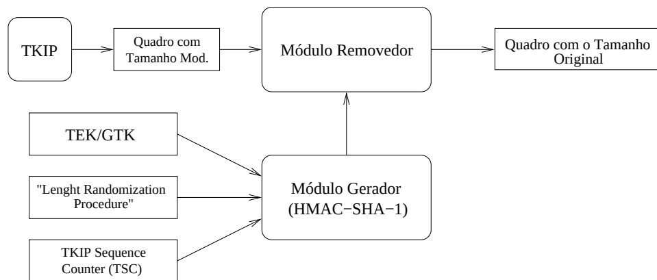
Figura 4.3 Procedimento de Remoção
