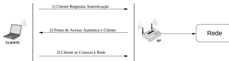
Figura 2.1 Autenticação por Sistema Aberto ( Open System )
