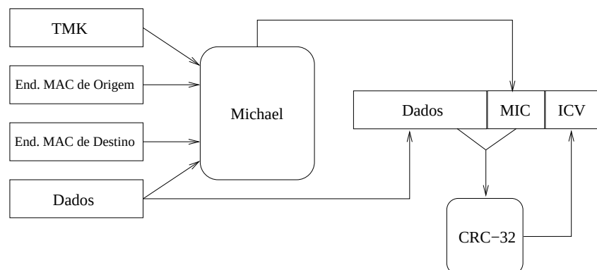
Figura 3.3 Integridade WPA
