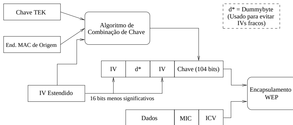
Figura 3.4 Confidência WPA
