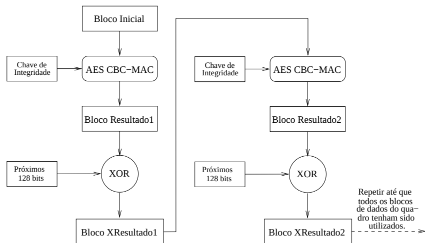
Figura 3.5 Integridade WPA2
