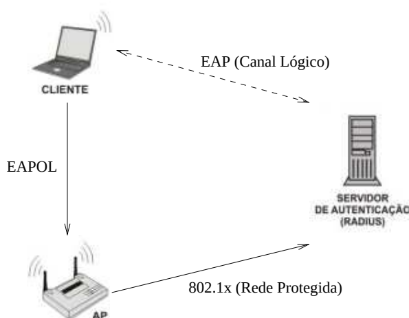
Figura 3.1 Esquema de protocolos do WPA corporativo
