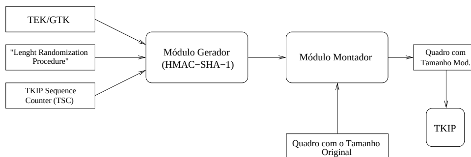
Figura 4.2 Procedimento de Inserção
