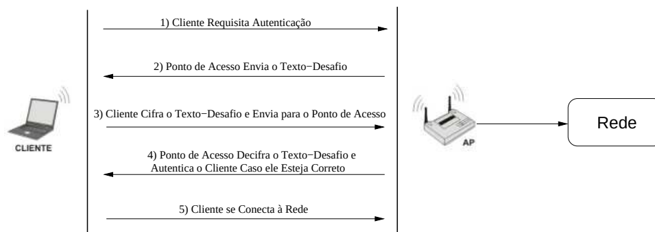
Figura 2.2 Autenticação por Chave Compartilhada ( Shared Key )
