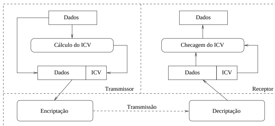
Figura 2.3 Checagem de Integridade no Protocolo WEP
