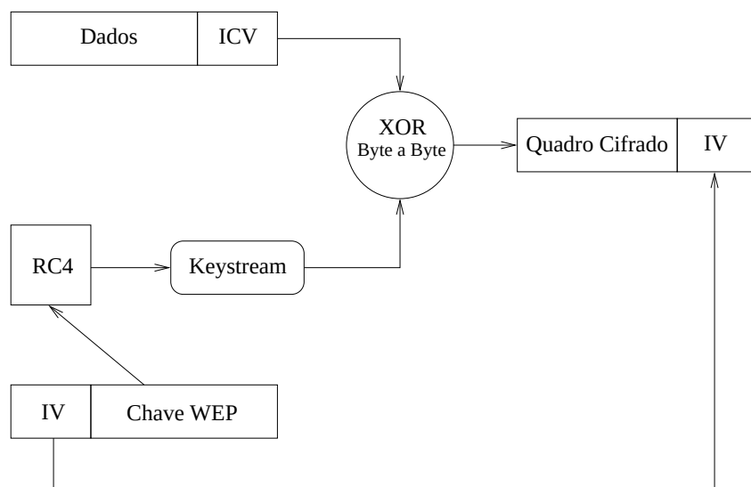
Figura 2.4 Esquema de criptografia do WEP
