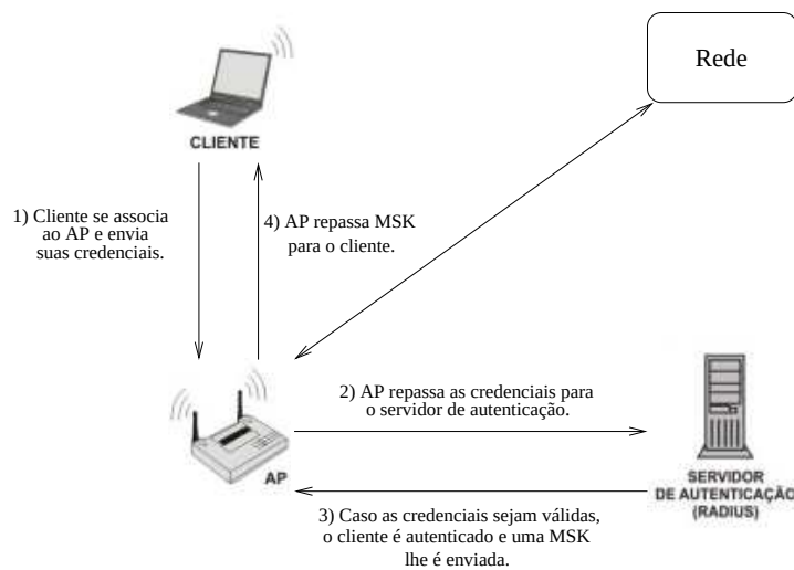
Figura 3.2 Autenticação WPA corporativo
