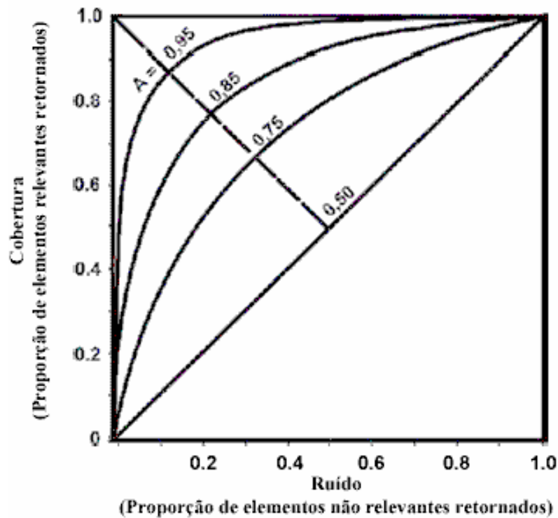
Figura 3.4 - Exemplos de curvas ROC da cobertura vs. ruído. A área A sob a curva indica a separação entre os elementos relevantes dos não relevantes.
