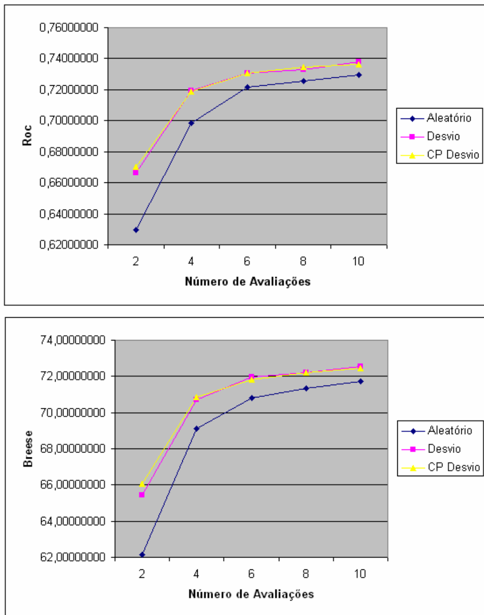
Figura 5.6 - Comparação entre Desvio isoladamente e o Desvio combinado com a Popularidade.
