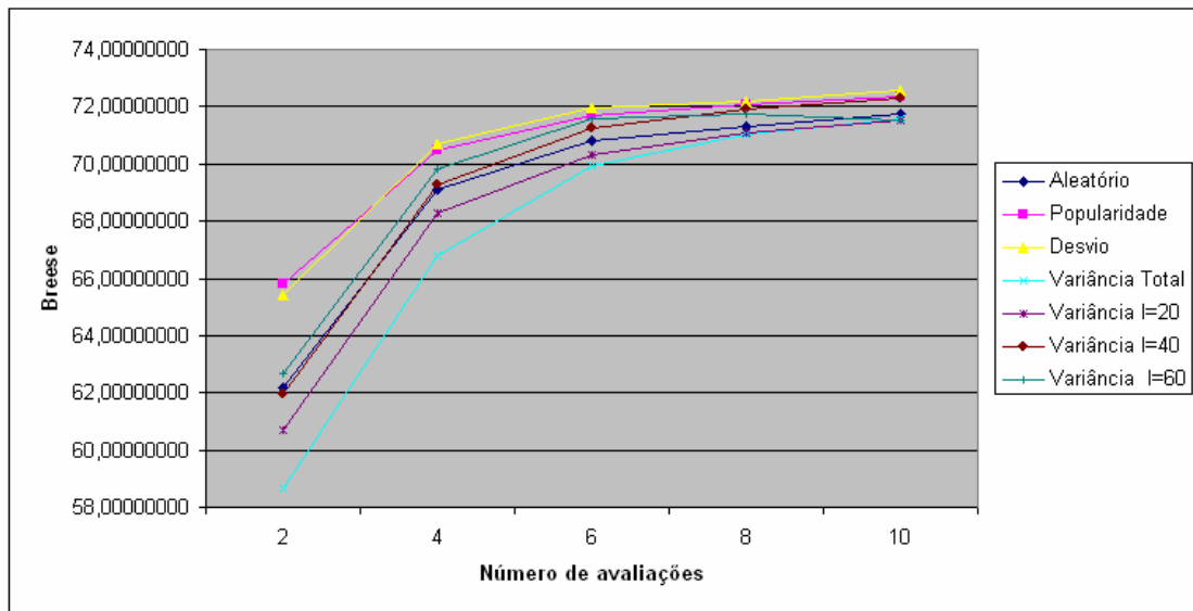
Figura 5.4 - Gráficos da performance das predições usando perfil do usuário formado pelos itens selecionados com os critérios isolados.
