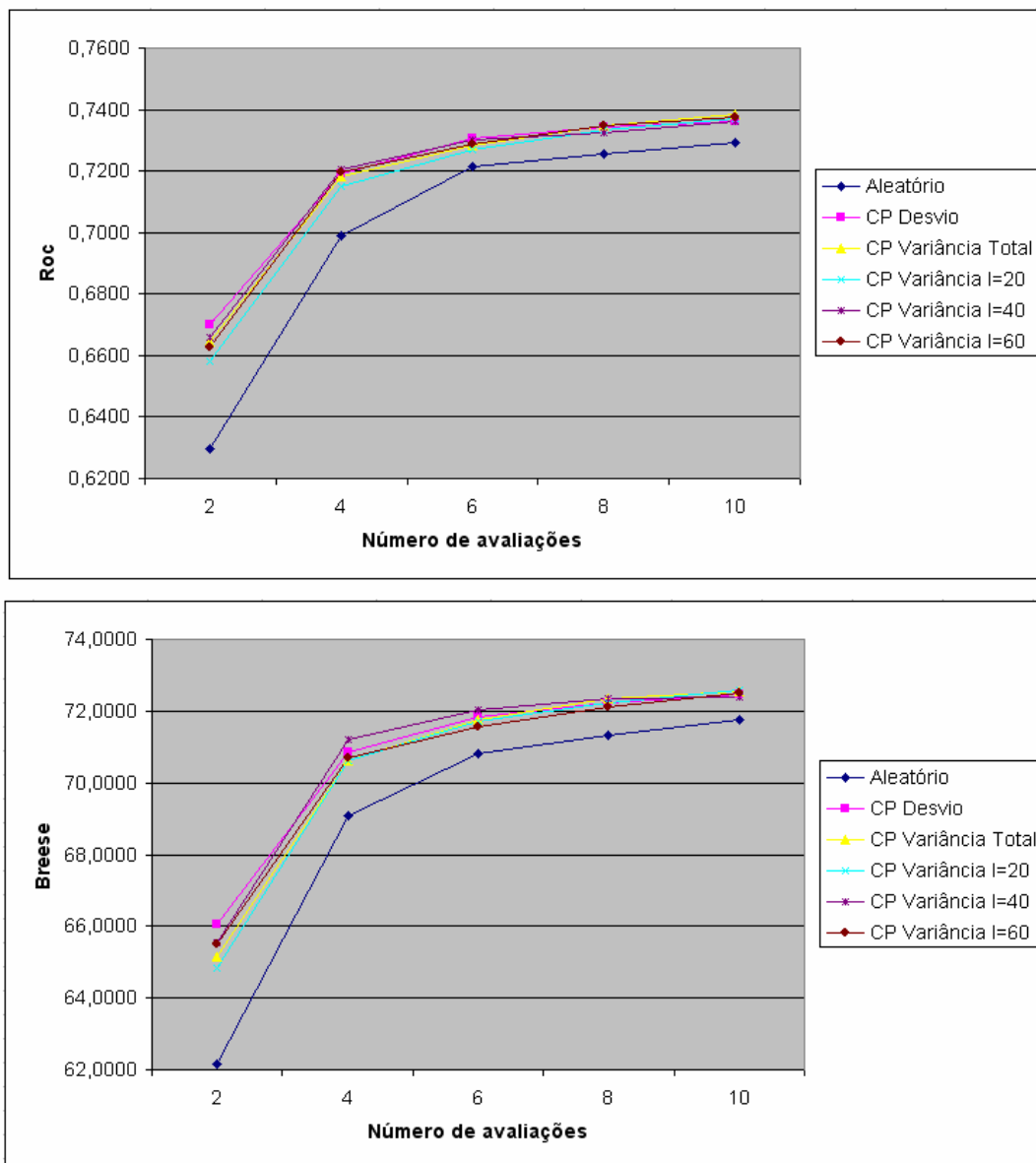
Figura 5.5 - Gráficos da performance das predições usando perfil do usuário formado pelos itens selecionados com os critérios combinados.
