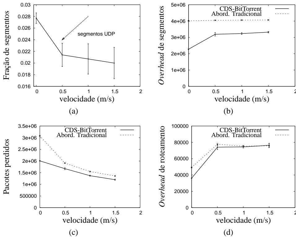
Figura 6. Cenário com Mobilidade: (a) Fração de segmentos (b) Overhead de segmentos (c) Pacotes perdidos (d) Overhead de roteamento
