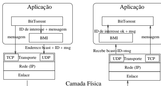
Figura 2. Pilha de protocolos com a interface BMI
